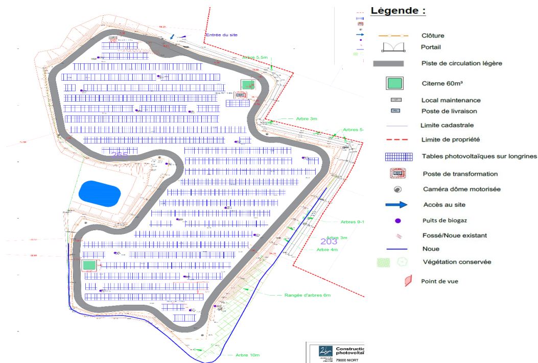
Plan masse du projet – extrait étude d'impact page 30
